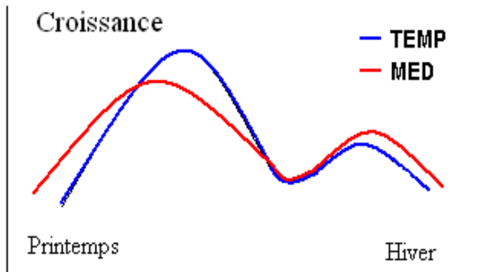
Figure 9—Schéma explicatif de la distribution annuelle de la vitesse de croissance de populations de luzerne ou de fétuque d'origines méditerranéennes (rouge) ou tempérées (bleu). Source : Gastal et al., 2015 .
