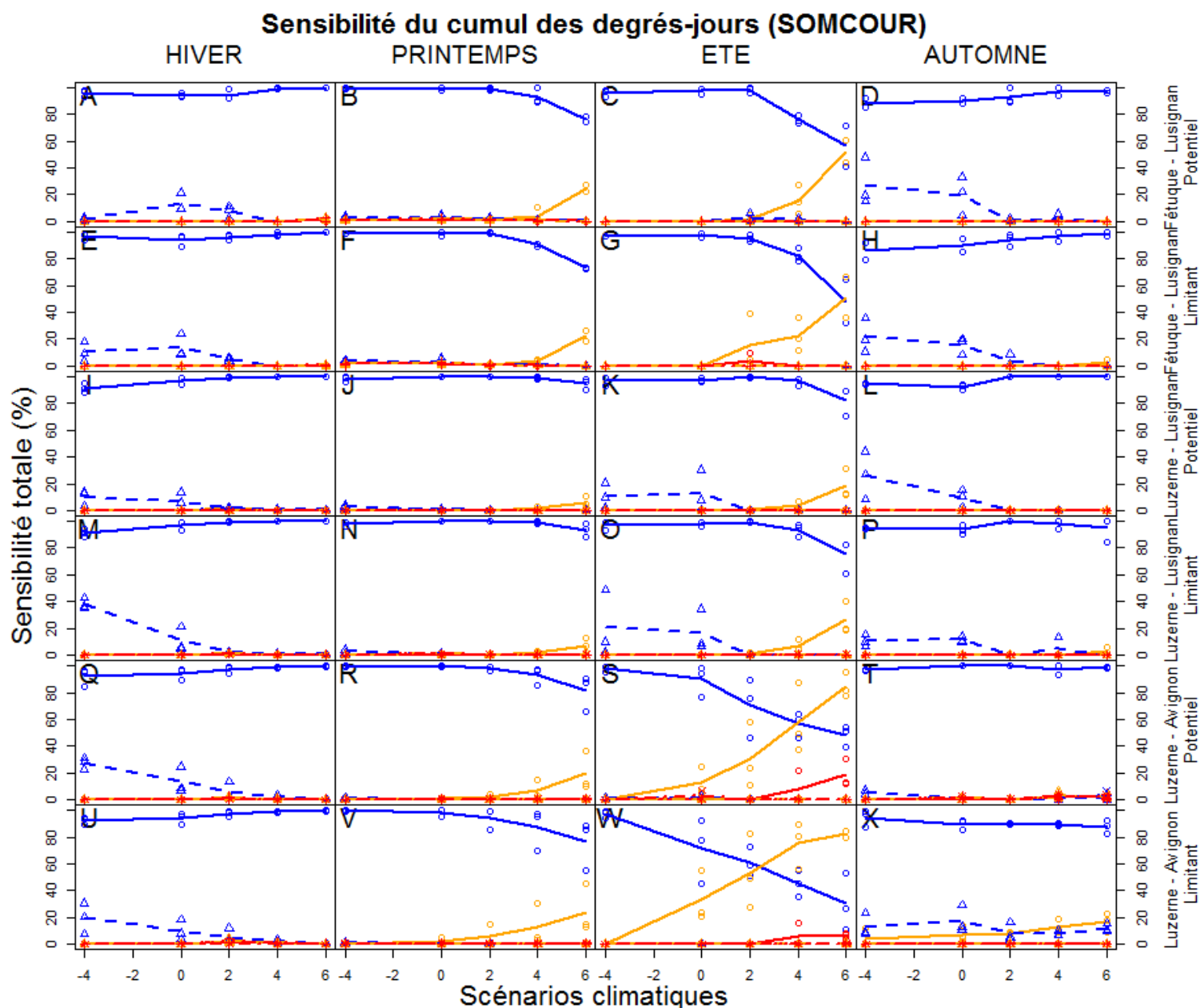
Figure 44—Sensibilité totale saisonnière (% , hiver 1 ère colonne, printemps 2 ème colonne, été 3 ème colonne et automne 4 ème colonne) du cumul de degrés-jours (SOMCOUR) pour trois années contrastées issues de différents scénarios climatiques (allant de -4 à +6^{\circ}\text{C} ) dans deux zones climatiques (Lusignan, tempérée pour les deux espèces ; Avignon, Méditerranéenne, pour la luzerne) et sous deux conditions de culture (potentielle ou limitante).
