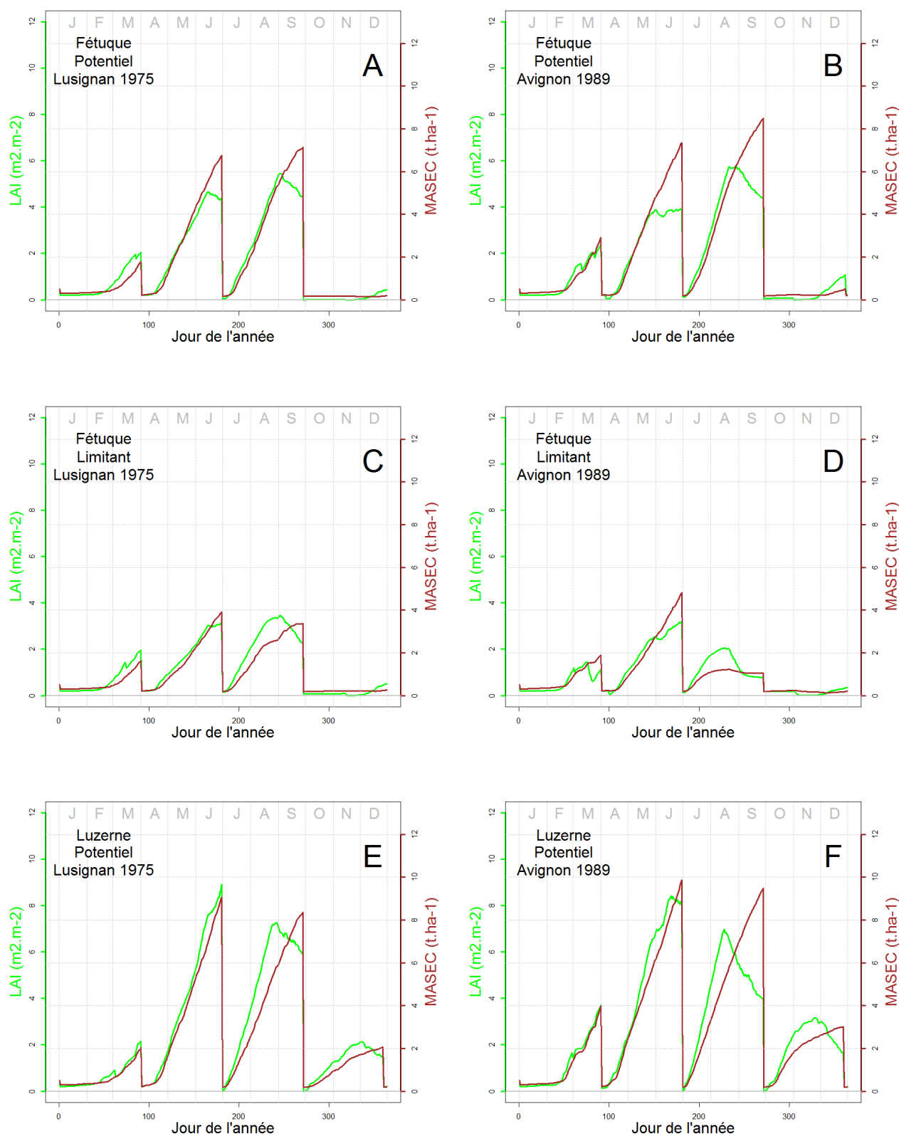
Figure 42—Illustrations de quelques sorties de simulations d'indices foliaires (LAI, \text{m}^2.\text{m}^{-2} , courbe verte ) et de matières sèches aériennes totales (MASEC, \text{t}.\text{ha}^{-1} , courbe rouge ) pour un scénario climatique actuel pour une fétuque à Lusignan en conditions potentielles ou limitantes (A et C respectivement) ou à Avignon en conditions potentielles ou limitantes (B et D respectivement). Les simulations de la Luzerne à Avignon en conditions potentielles sont données respectivement en E et F. Les simulations sont effectuées pour des années climatiques moyennes pour chaque zone climatique (1975 pour Lusignan et 1989 pour Avignon, Tableau 11 ).
