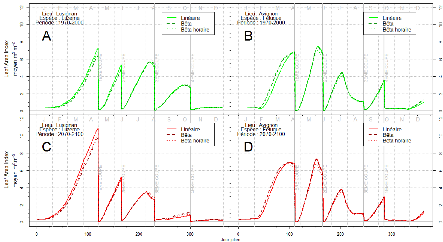
Figure 61 - Evolution du Leaf Area Index ( \text{m}^2 \cdot \text{m}^{-2} , moyenne sur 30 ans) du modèle « linéaire » et « bêta » (A et B) ou « bêta horaire » (C et D) sur deux périodes (1970-2000, verts ; 2070-2100, rouges ) de la fétuque à Avignon (A et C) et de la luzerne à Lusignan (B et D).
