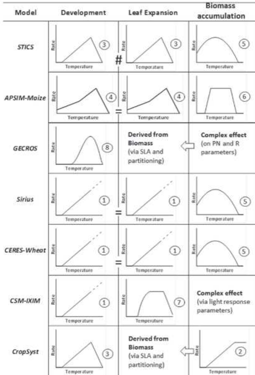
Figure 21—Formalismes de réponse à la température du développement, de la croissance foliaire et de l'accumulation de biomasse pour différents modèles du culture à la suite de l'étude bibliographique de Parent et Tardieu (2014) . Différents formalismes mathématiques simplifiés sont représentés : 1) des fonctions linéaires simples, 2) des fonctions bilinéaires à plateau, 3) des fonctions bilinéaires, 4) des fonctions tri-linéaires, 5) des fonctions hyperboliques, 6) des fonctions trapézoïdes, 7) des fonctions de type « bêta dérivées ».
