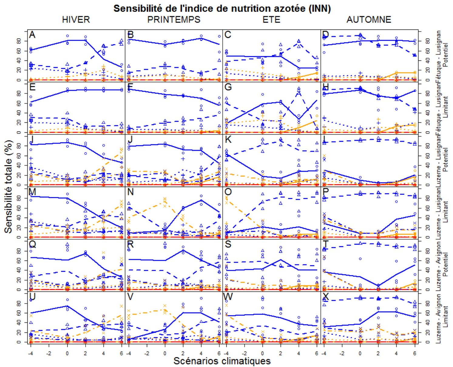
Figure 46—Sensibilité totale saisonnière (% , hiver 1 ère colonne, printemps 2 ème colonne, été 3 ème colonne et automne 4 ème colonne) de l'indice de nutrition azotée (INN) pour trois années contrastées issues de différents scénarios climatiques (allant de -4 à +6^{\circ}\text{C} ) dans deux zones climatiques (Lusignan, tempérée pour les deux espèces ; Avignon, Méditerranéenne, pour la luzerne) et sous deux conditions de culture (potentielle ou limitante).
