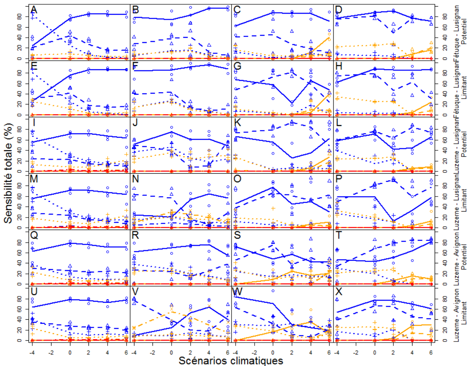
Figure 46—Sensibilité totale saisonnière (% , hiver 1 ère colonne, printemps 2 ème colonne, été 3 ème colonne et automne 4 ème colonne) de la matière sèche aérienne totale (MASEC) pour trois années contrastées issues de différents scénarios climatiques (allant de -4 à +6^{\circ}\text{C} ) dans deux zones climatiques (Lusignan, tempérée pour les deux espèces ; Avignon, Méditerranéenne, pour la luzerne) et sous deux conditions de culture (potentielle ou limitante).
