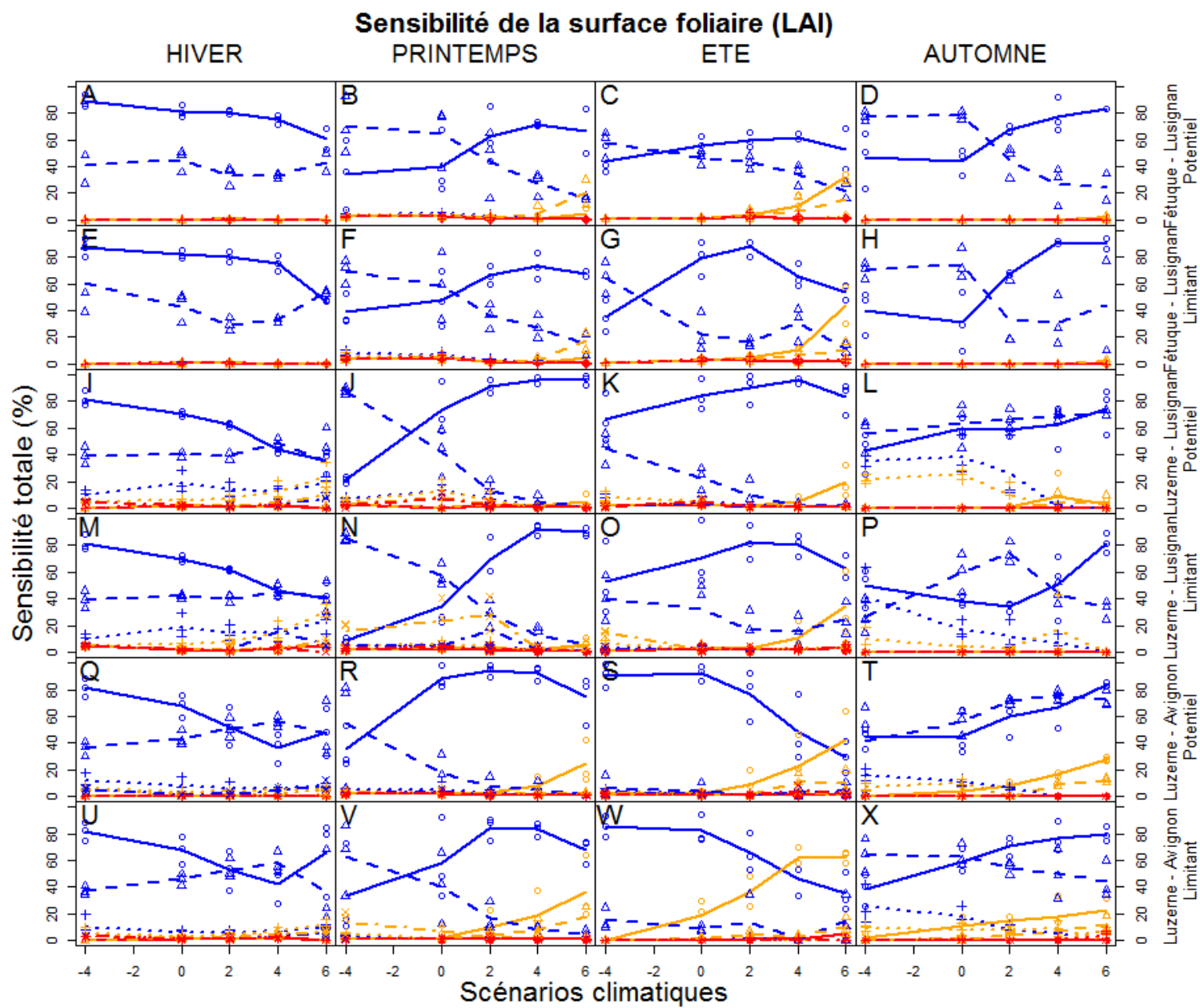
Figure 45—Sensibilité totale saisonnière (% , hiver 1 ère colonne, printemps 2 ème colonne, été 3 ème colonne et automne 4 ème colonne) de l'indice foliaire (LAI) pour trois années contrastées issues de différents scénarios climatiques (allant de -4 à +6^{\circ}\text{C} ) dans deux zones climatiques (Lusignan, tempérée pour les deux espèces ; Avignon, Méditerranéenne, pour la luzerne) et sous deux conditions de culture (potentielle ou limitante).
