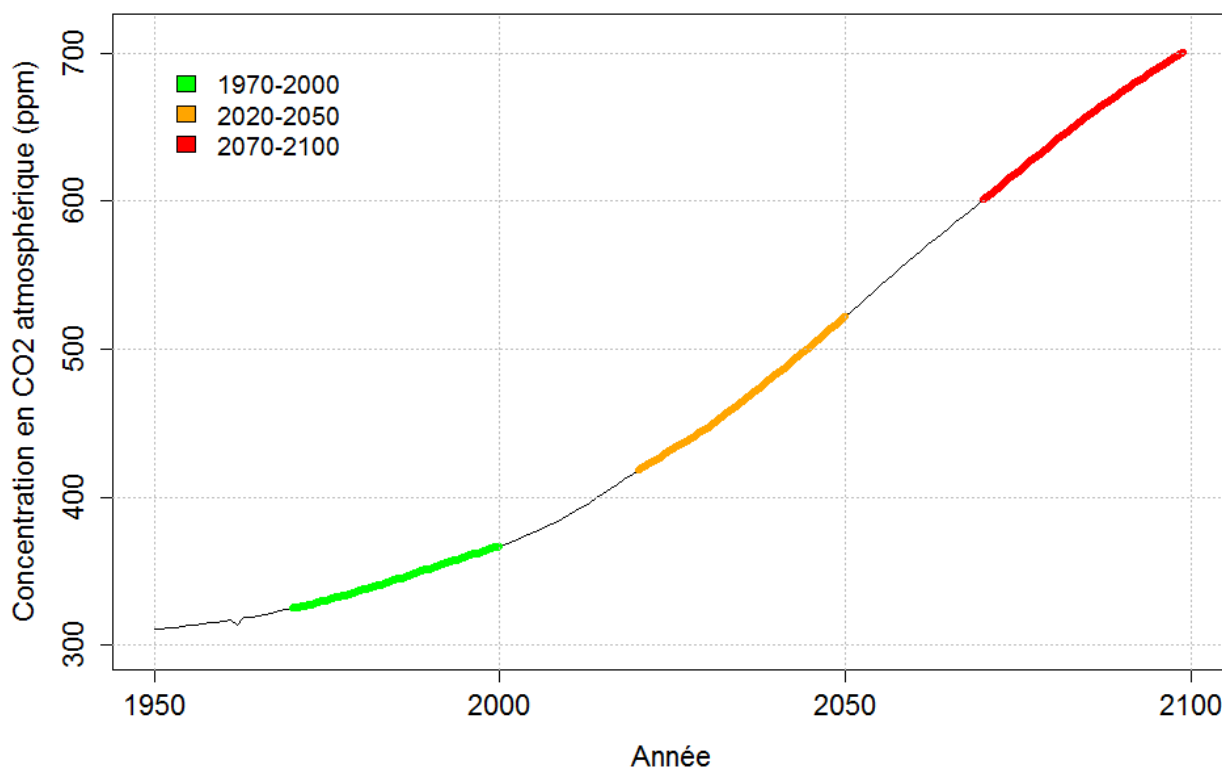
Figure 56 - Evolution de la concentration en Co2 atmosphérique pour les deux sites entre 1950 et 2100 entre le passé proche (1970-2000, vert ), le futur proche (2020-2050, orange ) et le futur lointain (2070-2100, rouge ).
