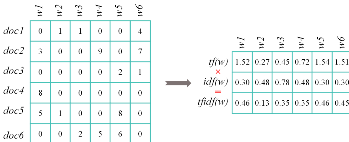
FIGURE 3.3 – Principe de calcul du TF-IDF. La matrice de gauche représente les occurrences des différents mots w pour chaque document doc .
