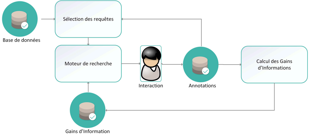
FIGURE 5.6 – Schéma général de notre approche adaptative.
