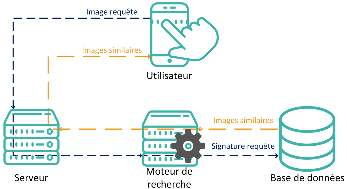
FIGURE 1.3 – Système de recherche d'images par similarité.
