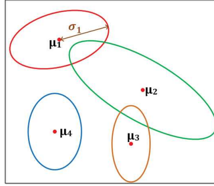
Figure 1.8: Illustration des différentes hypothèses de l'algorithme GMM.
