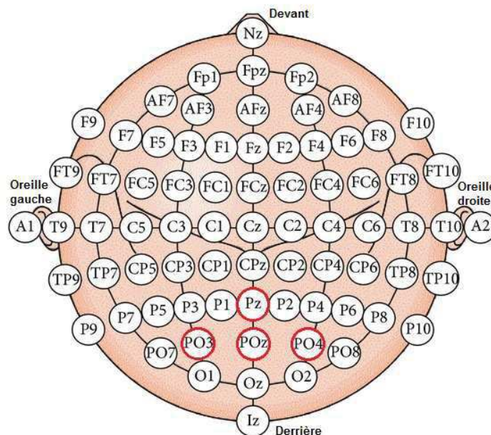
Figure 4.10: Positionnement des électrodes dans le système international 10-20 [Ele ]. Les 4 potentiels que nous avons utilisées sont entourés en rouge.
