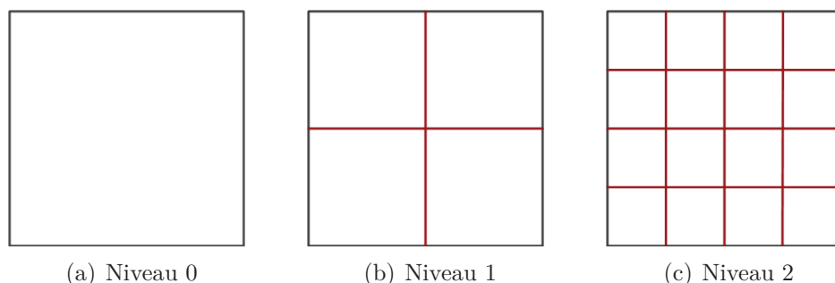
Figure 1.10: Illustration de la pyramide spatiale proposée par Lazebnik et al. [Lazebnik 06].
