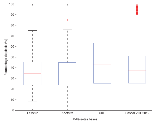
(d) FAST
