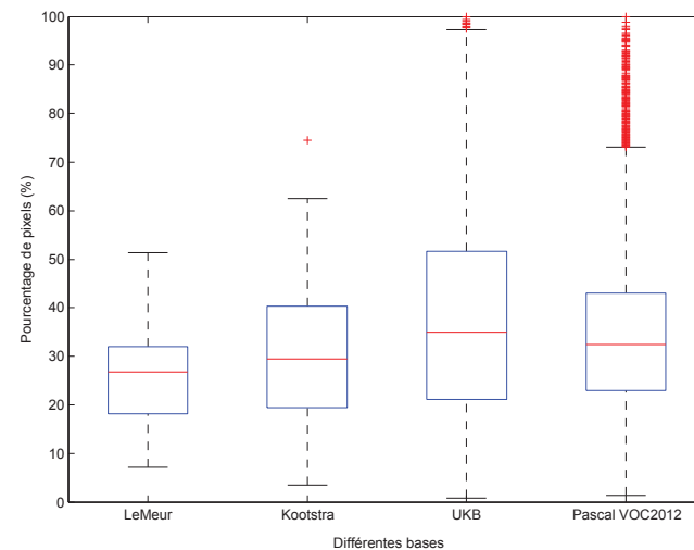
(b) Harris-Laplace
