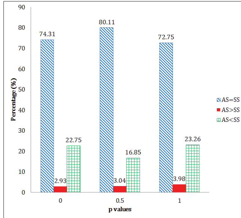
Figure 2.10: Étude du rang des images ressemblantes en pondérant les vecteurs de descripteurs par la saillance du point décrit. La notation AS signifie "Avec ondération par la saillance" et SS "Sans pondération".
