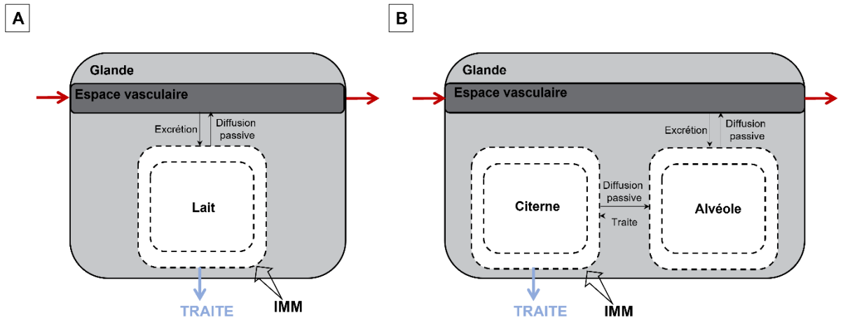
Figure 12: Modèles de la glande mammaire à 1 compartiment (A) ou 2 compartiments (B) développés par Li.
